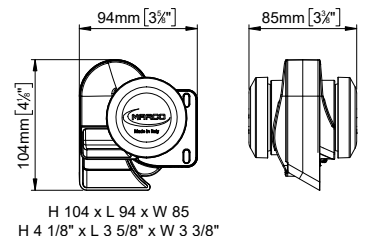
COMPRESSORE COMPRESSOR
